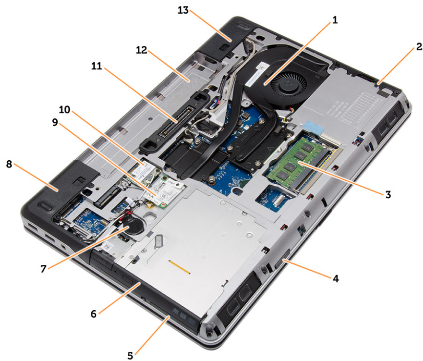
圖 1. 後視圖 — 後蓋已卸下
